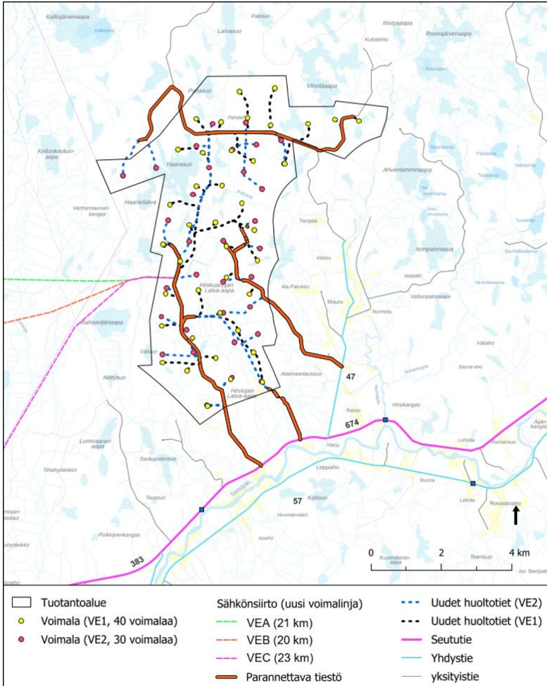
Kuva 9.13 Tuotantoalueen suunnitellut sisääntulotiet sekä olemassa olevat parannettavat tieyhteydet ja uudet huoltotiet voimaloiden välillä.
