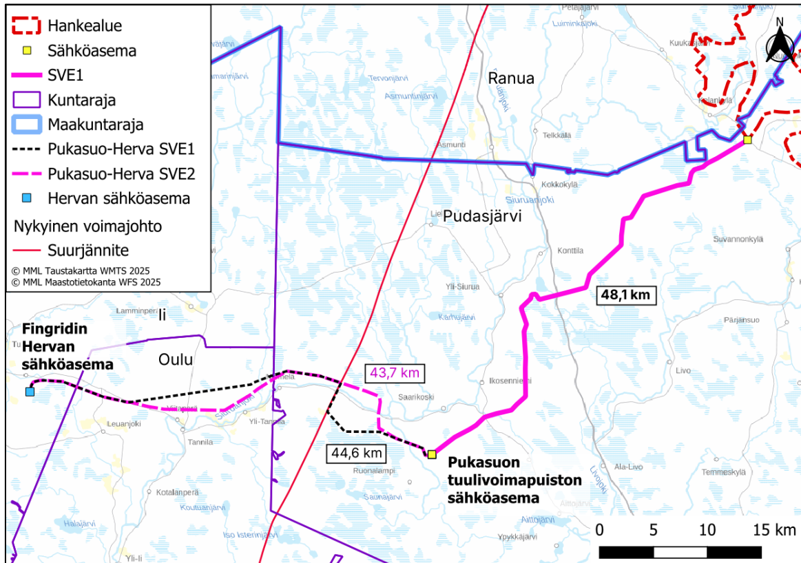
Kuva 4 Reitin SVE1 liittyminen Pukasuon tuulivoimapuiston sähköasemalta Fingridin Hervan sähköasemalle lihin.
